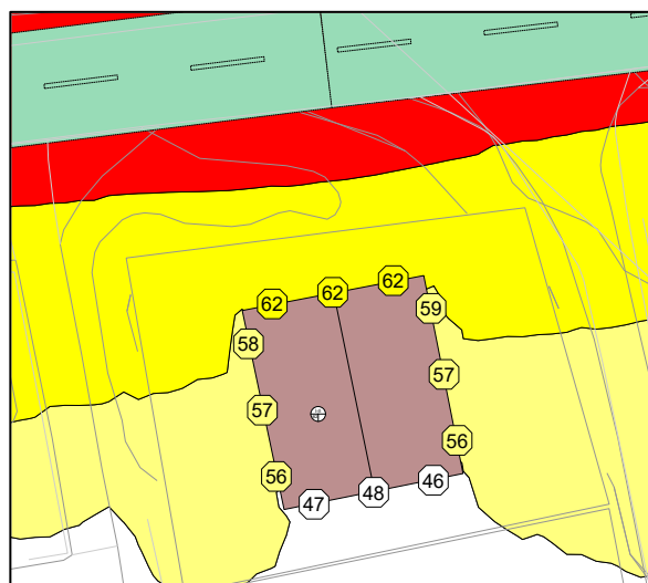
Figur 4-4: Beregnede fasadepunkter i 2. etg. for fremtidig situasjon uten tiltak.
