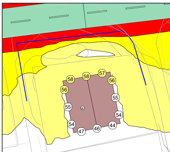
Figur 4-9: Fremtidig situasjon med støyskjem på 2,5 meter langs kanten av tomten i nord og deler av vest og øst. Beregnede fasadepunkter i 2. etg.
