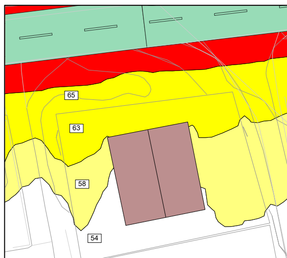
Figur 4-6: Støysone for fremtidig situasjon uten tiltak beregnet på 1,5 meters høyde og 1x1 meters oppløsning.
