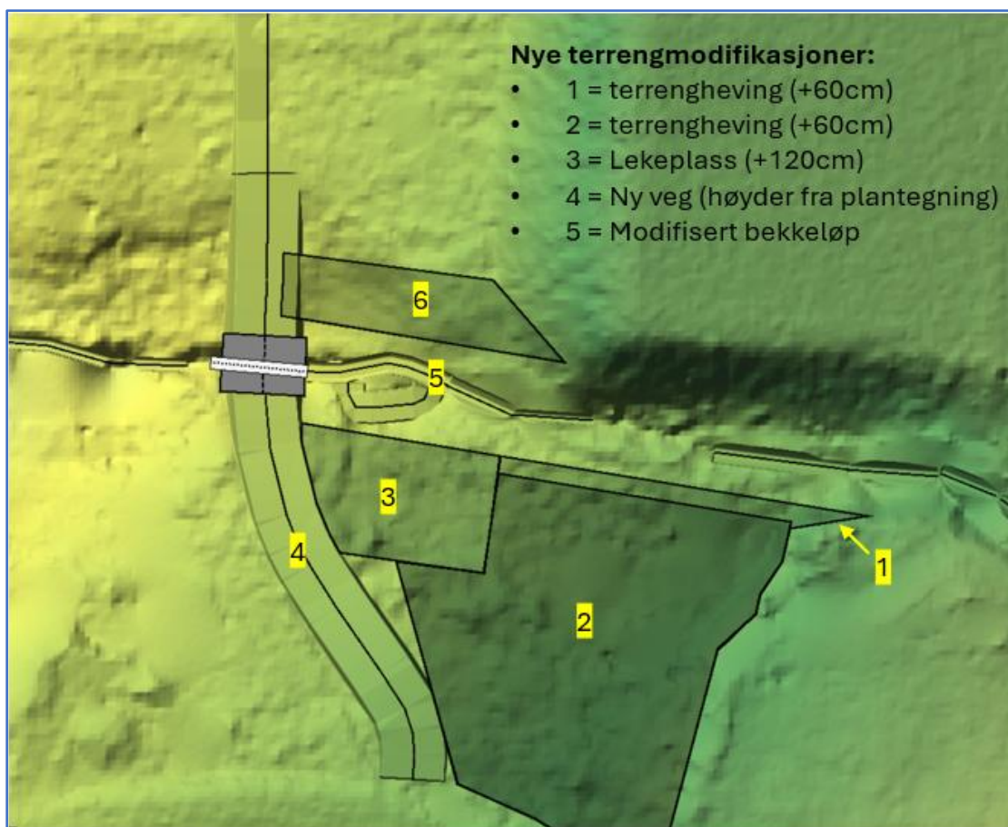
Figur 2. Visualisering av terrengheving i modellen. Røde linjer viser eiendomsgrenser, sorte stiplede linjer er høydekoter.
