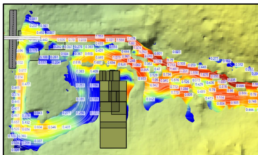
Vedlegg 9. Flomsoner nederst i elveløpet. Figuren viser vannhastigheter Q-200 flomsituasjon (med klimapåslag).
