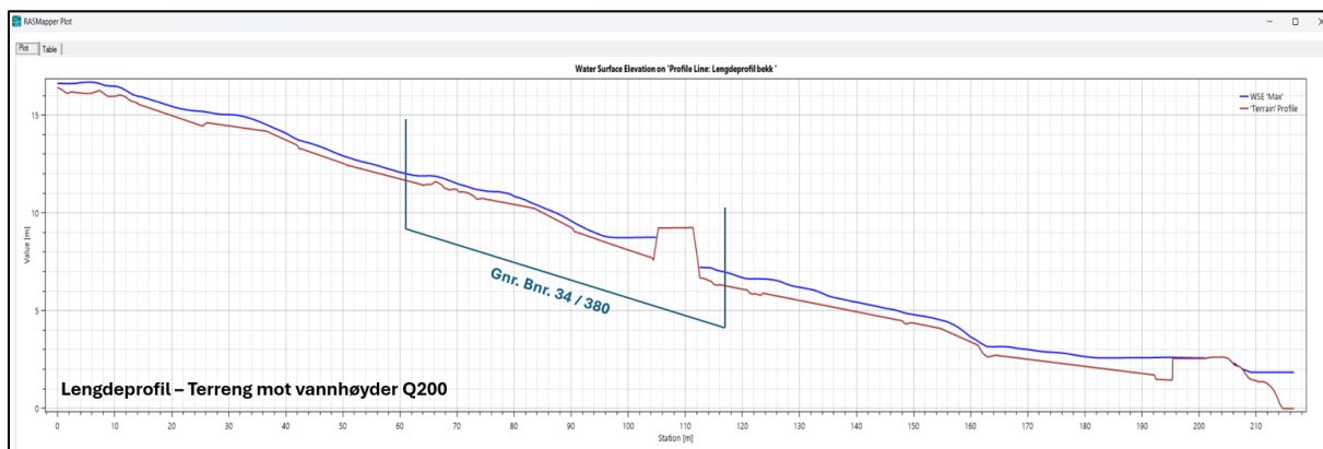
Vedlegg 4. Lengdeprofil - Vannhøyder mot terreng langs elveprofilen.
