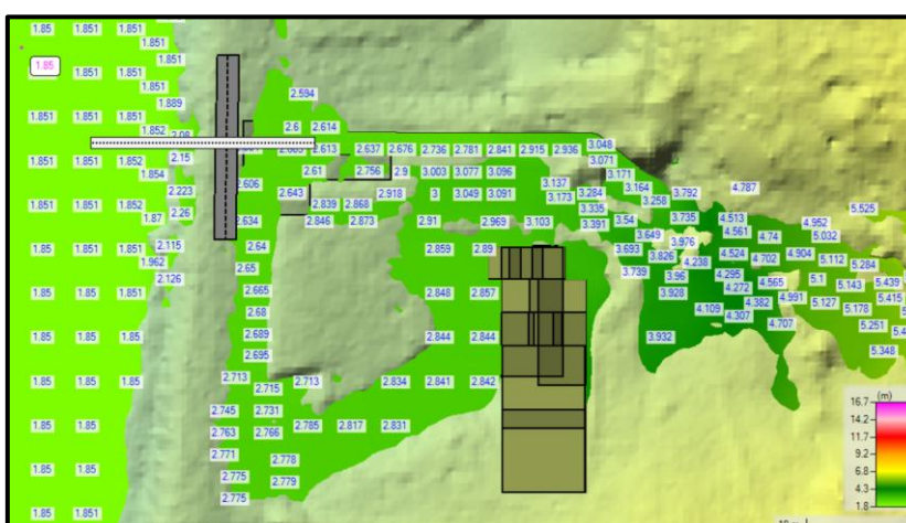
Vedlegg 10. Flomsoner nederst i elveløpet. Figuren viser vannhøyder Q-200 flomsituasjon (med klimapåslag).
