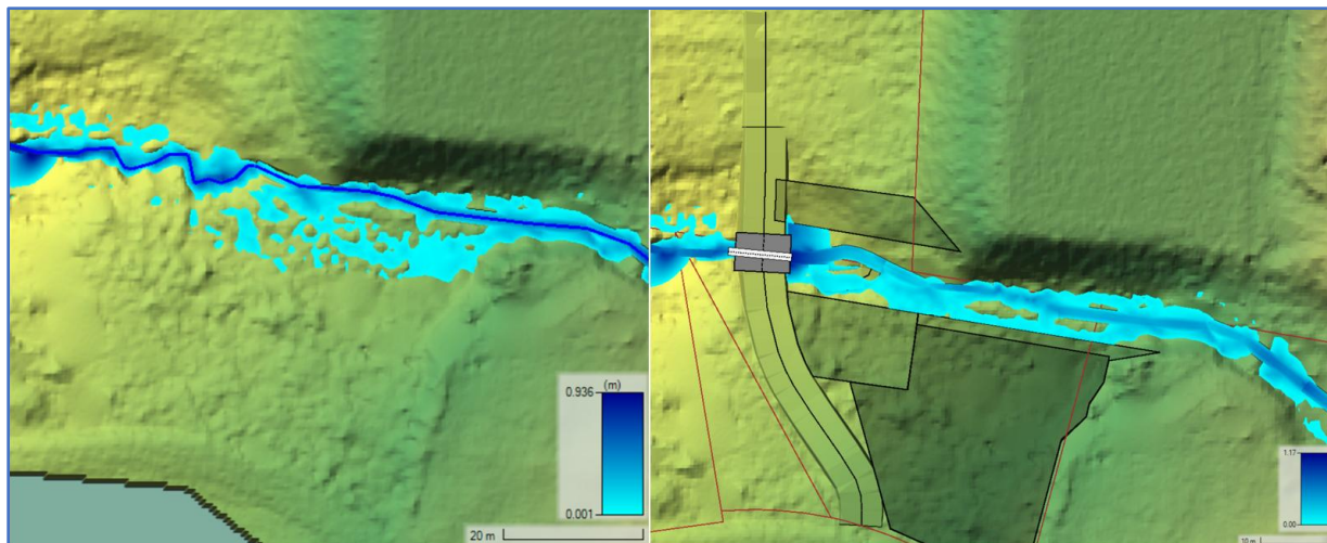
Figur 5. Vanndybder ved Q200 før tiltak (venstre) og etter tiltak (høyre).
