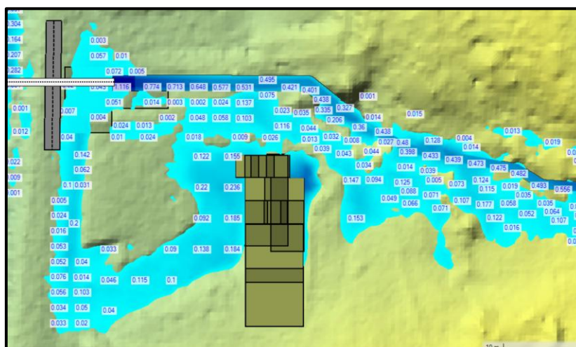
Vedlegg 8. Flomsoner nederst i elveløpet. Figuren viser vanndybder Q-200 flomsituasjon (med klimapåslag).
